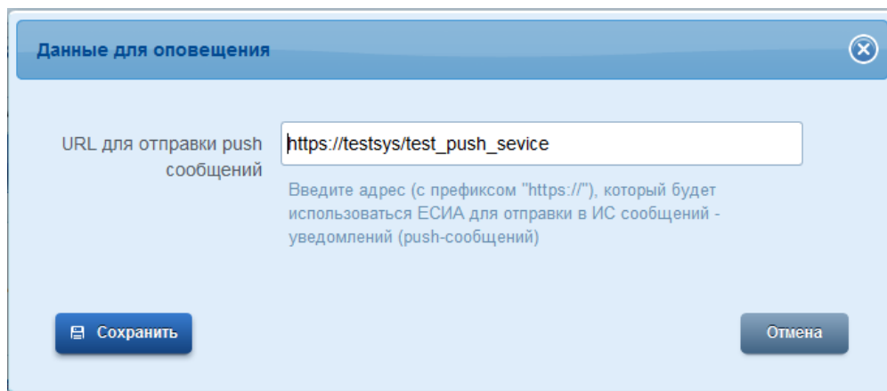
Рисунок 31 – Ввод или редактирование URL-адреса REST-сервиса ИС организации для приёма уведомлений о событиях платформы согласий ЕСИА
