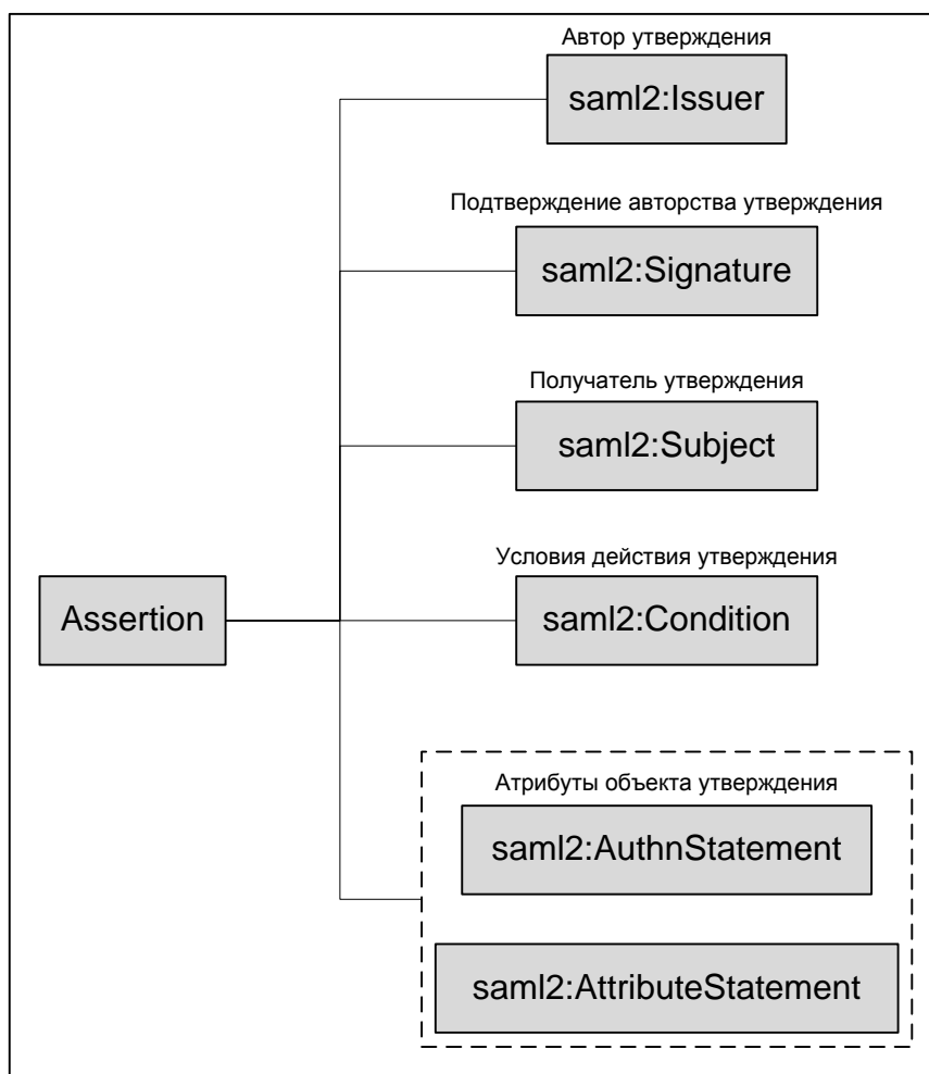
Рисунок 8 – Структура AuthnResponse
