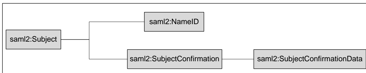
Рисунок 9 – Структура saml2:Subject
