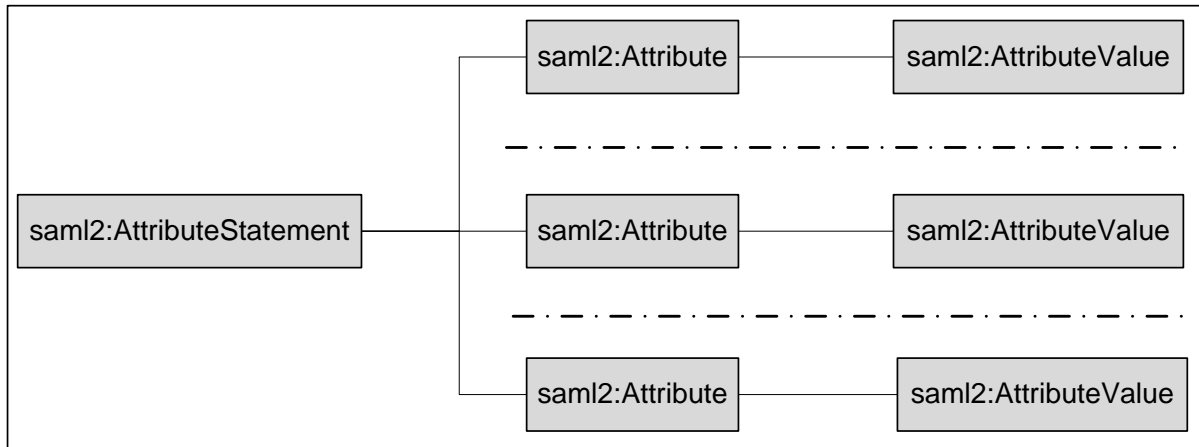
Рисунок 10 – Структура saml2:AttributeStatement
