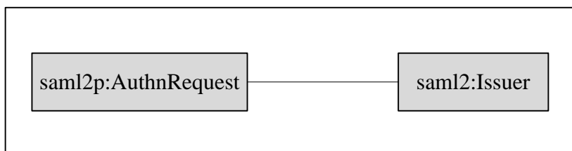
Рисунок 7 – Структура AuthnRequest
