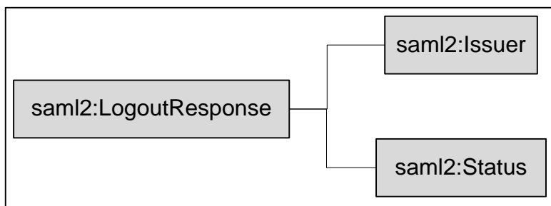
Рисунок 12 – Структура LogoutResponse
