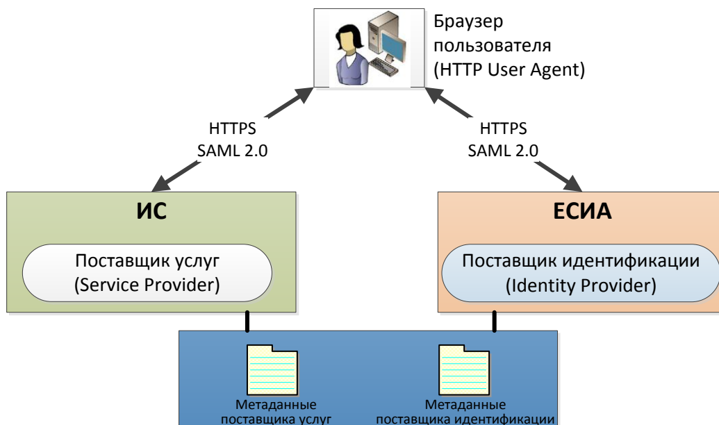
Рисунок 1 – Схема взаимодействия ИС с ЕСИА с целью идентификации и аутентификации с использованием стандарта SAML 2.0
