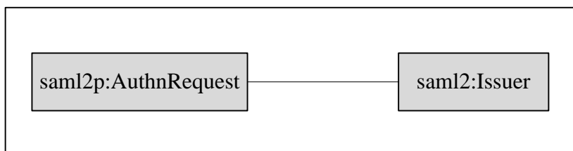
Рисунок 7 – Структура AuthnRequest
