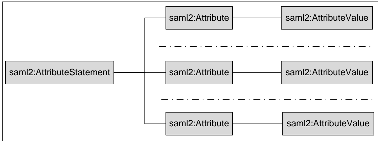
Рисунок 10 – Структура saml2:AttributeStatement
