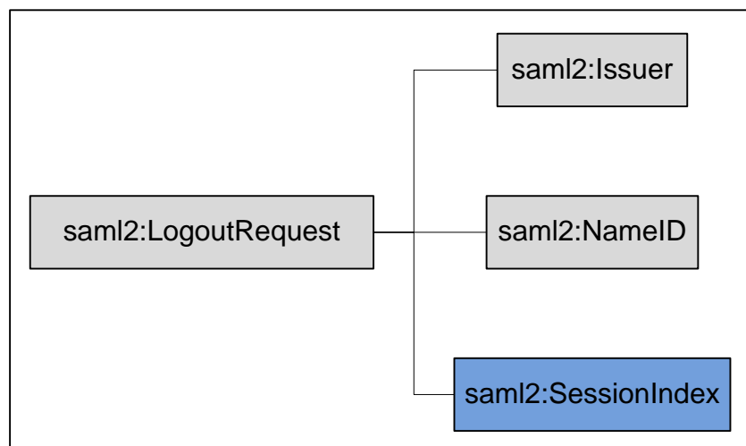
Рисунок 11 – Структура LogoutRequest
