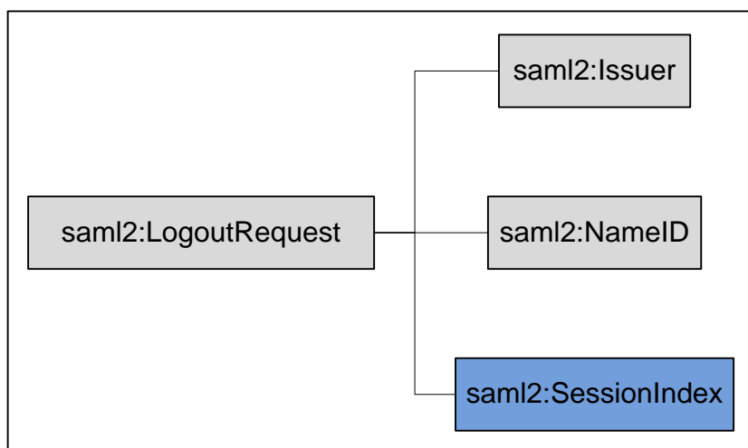
Рисунок 11 – Структура LogoutRequest
