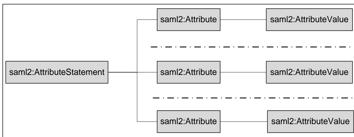
Рисунок 10 – Структура saml2:AttributeStatement
