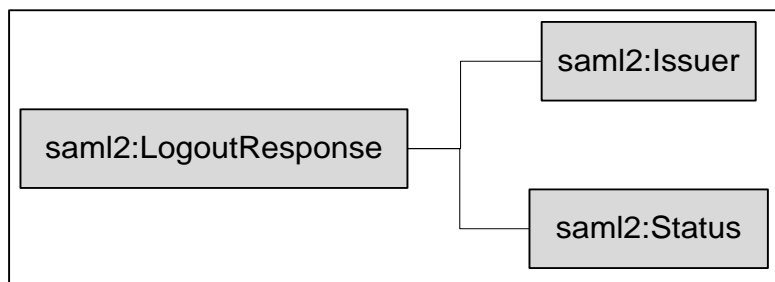
Рисунок 12 – Структура LogoutResponse
